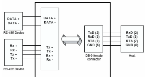
ADAM-4520I Converter Module
