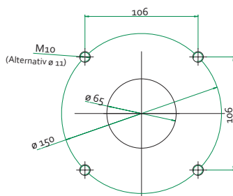
HLT Aufsatzgelenk / Setup joint Art. Nr. / Part No.: 40101-01
